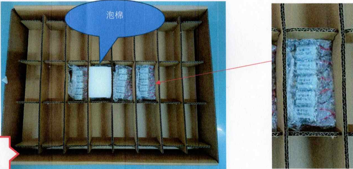
图一，每 5 个组件用 1 个气泡袋包装，每格 1 袋，每格 5pcs，每袋组件上方放一个切好的泡棉（每个泡棉切为 3 块），每层 24 格，每层 120pcs，共 3 层，满箱 360pcs
