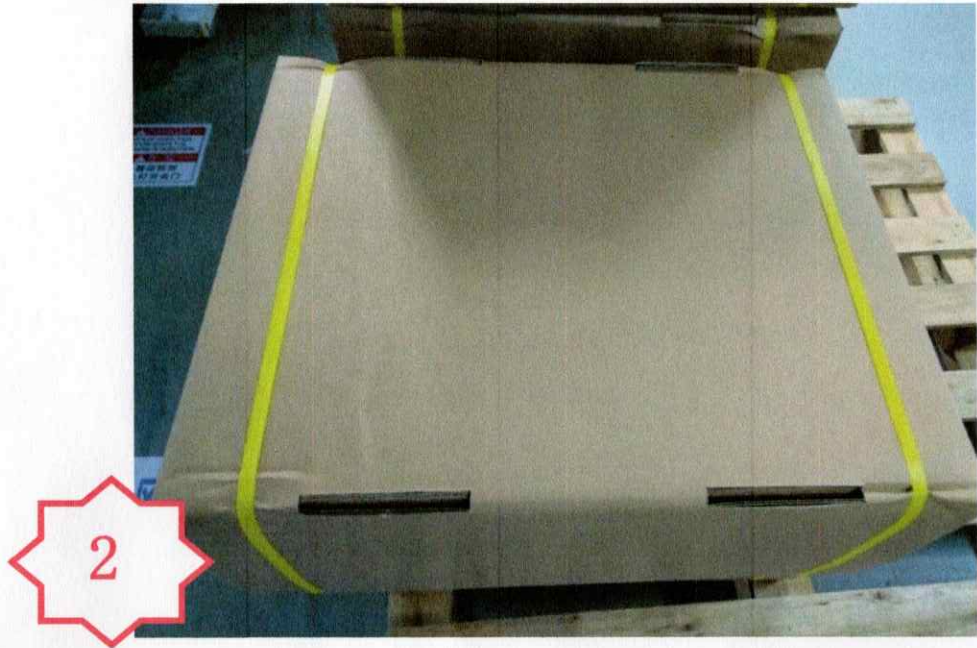
图二，确认 PA3214 无漏装后，将 22 的内箱与外箱配合并打包装带待出货
